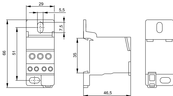
Рисунок 1 – Блоки распределительные РБД-80А
