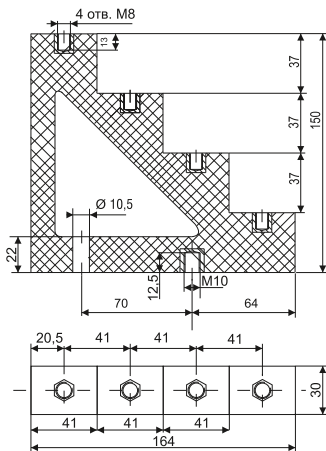
Рисунок 5. IC4-40
