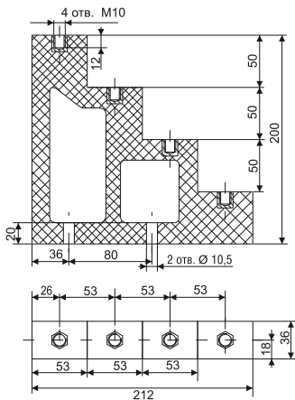
Рисунок 6. IC4-50
