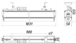
Рисунок 2 Светильник «L-trade II 45» с поворотным креплением
