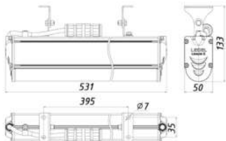
Рисунок 1 Светильник «L-trade II 20» с поворотным креплением
