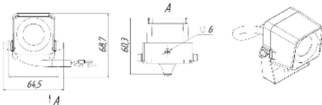
Рисунок 1 Светильник «L-mouse»
