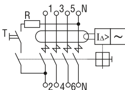
Рисунок 4 – Схема электрическая принципиальная четырехполюсных ВД
