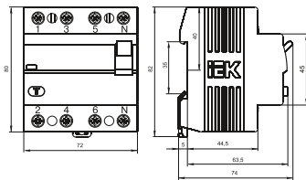
Рисунок 2 – Габаритные и установочные размеры четырехполюсных ВД
