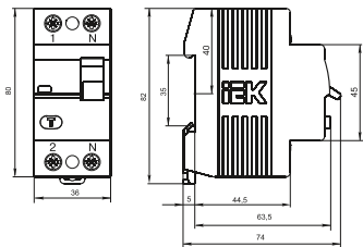
Рисунок 1 – Габаритные и установочные размеры двухполюсных ВД
