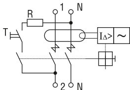
Рисунок 3 – Схема электрическая принципиальная двухполюсных ВД
