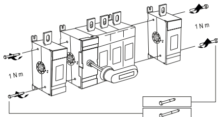
Рисунок 2. Схема установки дополнительного полюса
