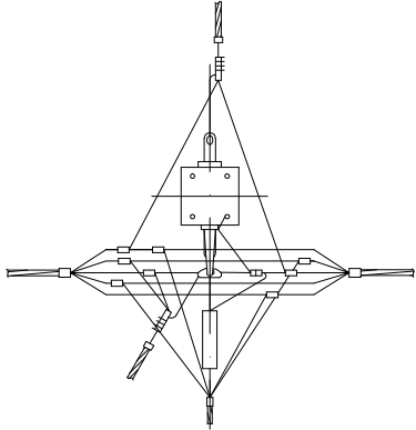
Схема ответвления к вводу в здания в две стороны 2х жил СИП
