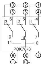
Рисунок 2. Схемы подключения
