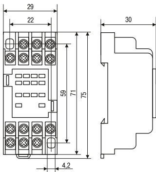
Рисунок 1. Габаритные размеры
