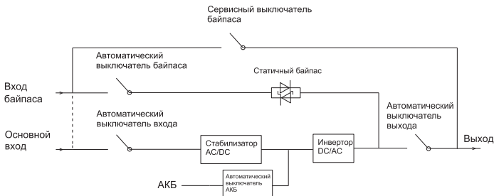
Рисунок 18 – Структура ИБП
