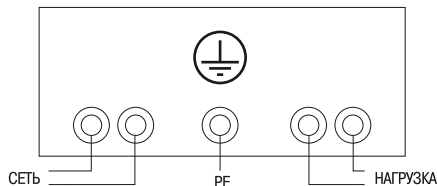
Рисунок 3. Схема подключения стабилизаторов мощностью 5 и 10 кВА
