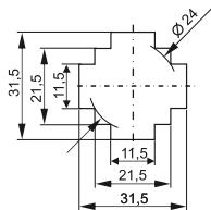
ТТИ-30 габарит 1
