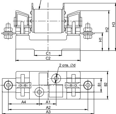
Рисунок 3 – ДП 35/37/39, габарит 1, 2 и 3 / Figure 3 – ДП 35/37/39, overall dimension 1, 2 and 3
