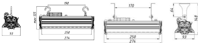
Рисунок 1 Общий вид светильника L-industry 30 Turbine, подвесное и поворотное крепление
