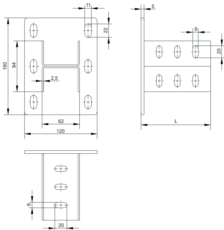
Рисунок 1 – Кронштейн потолочный двойной 110 / Figure 1 – Double ceiling bracket 110 / 1 сурет – Қосарлы төбе кронштейні 110
