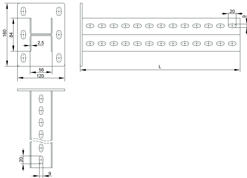
Рисунок 2 – Кронштейн потолочный двойной 400, 600 / Figure 2 – Double ceiling bracket 400, 600 / 2 сурет – Қосарлы төбе кронштейні 400, 600
