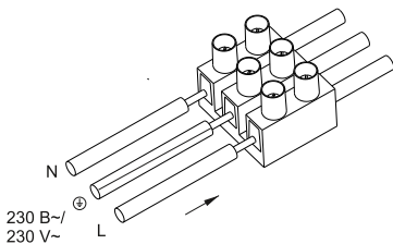
Рисунок А.1 – Подключение светильника/ Figure A.1 – Luminaire connection/ A.1-sýret – Shyraqdandy qosý/ Рисунок А.1 – Підключення світильника
