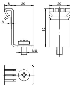
Рисунок 17 – Зажим балочный верт. 1-5мм с отгибом и винтом M6x10 HDZ / Figure 17 – Vertical beam clamp 1-5mm with bend and screw M6x10 HDZ / 17 сурет – Қайырмалы және M6x10 бұрандалы тік 1-5мм HDZ арқалықты қысқышы
