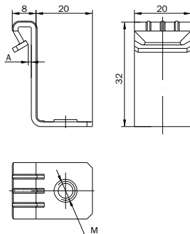
Рисунок 16 – Зажим балочный верт. 1-5мм с отгибом и резьбой HDZ / Figure 16 – Vertical beam clamp 1-5mm with bend and thread HDZ / 16 сурет – Қайырмалы және M6 бұрандалы тік 1-5мм HDZ арқалықты қысқышы
