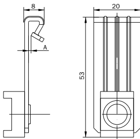
Рисунок 16 – Зажим балочный верт. 1-5мм с отгибом и резьбой HDZ / Figure 16 – Vertical beam clamp 1-5mm with bend and thread HDZ / 16 сурет – Қайырмалы және M6 бұрандалы тік 1-5мм HDZ арқалықты қысқышы
