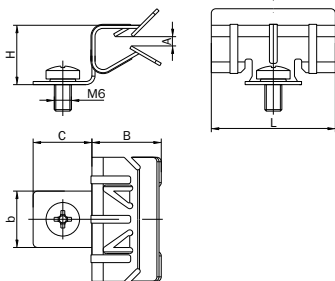
Рисунок 7 – Зажим балочный с отгибом и винтом M6x9 HDZ / Figure 7 – Beam clamp with bend and screw M6x9 HDZ / 7 сурет – Қайырмалы және M6x9 бұрандамалы HDZ арқалықты қысқышы
