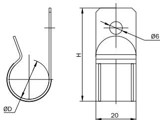
Рисунок 20 – Зажим балочный верт. 1-5мм под трубу HDZ / Figure 20 – Vertical beam clamp 1-5mm for pipe HDZ / 20 сурет – 20мм құбырға арналған 1-5мм тік HDZ арқалықты қысқышы
