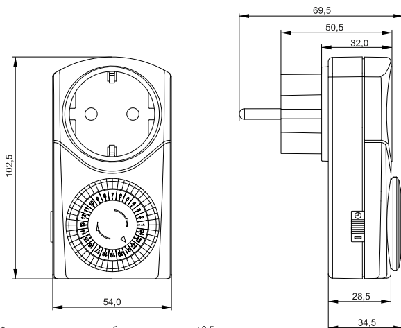
Рисунок 2 – PTM-1 Розетка-таймер
