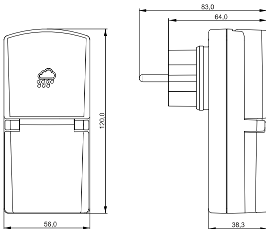
Рисунок 5 – PTM-4 Розетка-таймер
