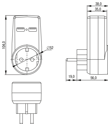
Рисунок 1 – Адаптер Т-01/01
