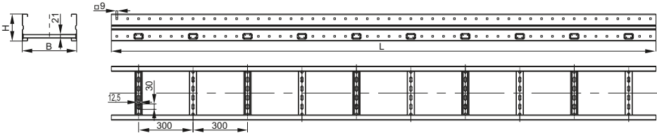
Рисунок 1 – Лоток лестничный LESTA 5H / Figure 1 – Ladder tray LESTA 5H / 1-сурет – LESTA 5H сатылы науасы
