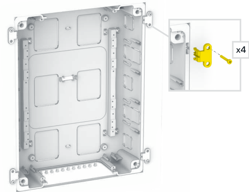
2.2 Крепление в полые стены ЩРВ-П Hollow wall mount
