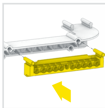
1.5.2 Крепление суппорта к кронштейну Support mount to the bracket
