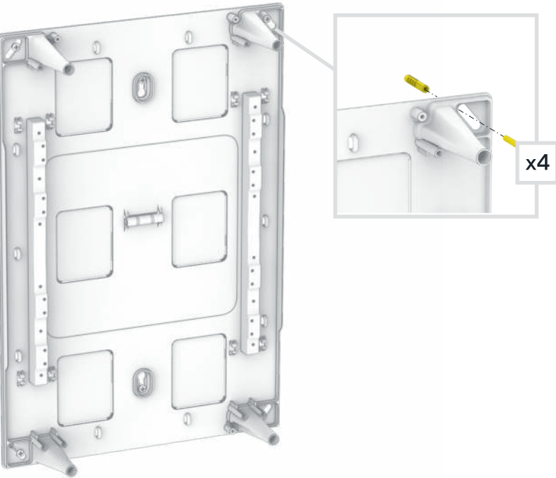
2.1 Крепление к стене ЩРН-П Wall mount
