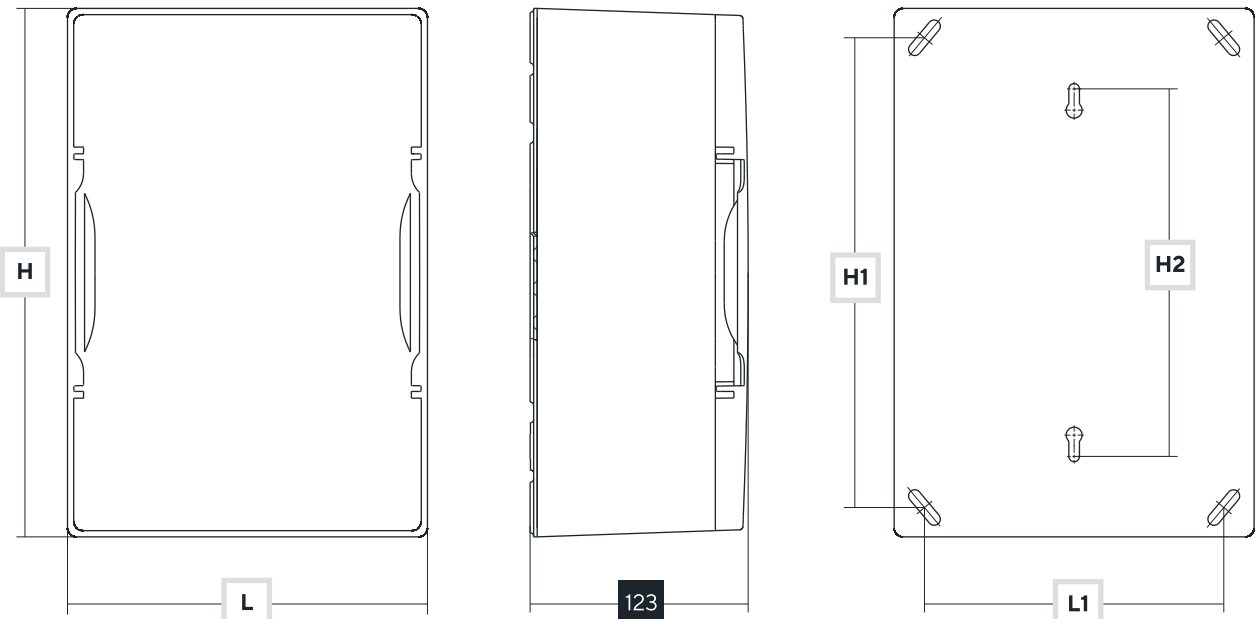
Крепление к стене ЩРН-П Wall mount
