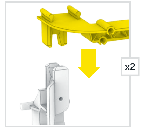
3.2 Крепление кронштейна к раме Bracket mount to the frame
