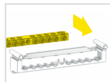
1.4 Крепление кронштейна к основанию** Bracket mount to the base**
