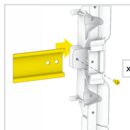
1.2.2 Установка DIN-реек* Installation of DIN rails*
