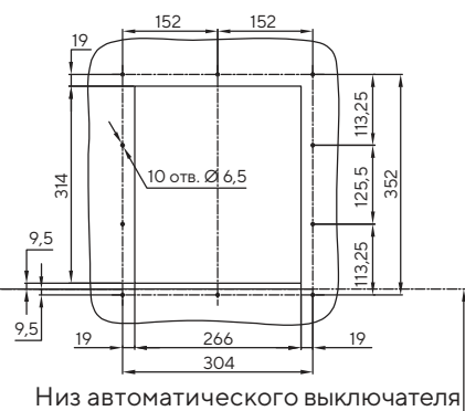
Расположение крепежных отверстий (вид снизу)
