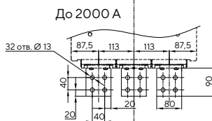
Вид Б (вертикальные выводы)
