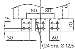
Вид А (горизонтальные выводы)
