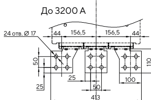
Вид А (горизонтальные выводы)
