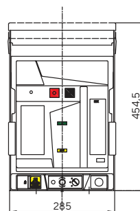
Вид спереди
