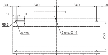
Расположение крепежных отверстий (вид снизу)
