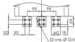
Вид Б (вертикальные выводы)
