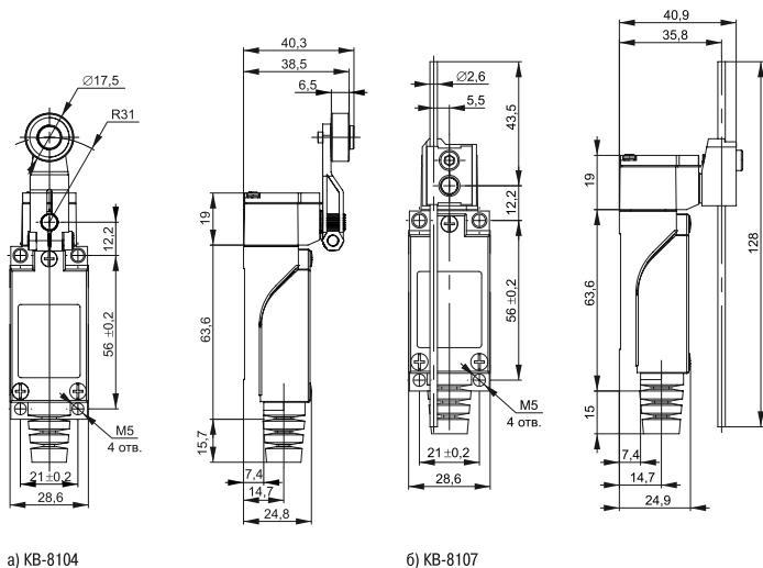
Рисунок Б.2 – Габаритные, установочные размеры концевых выключателей
