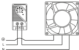
Рисунок 3 – Схема подключения
