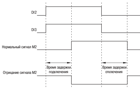
Рисунок 70 — Временная диаграмма работы внутреннего реле
