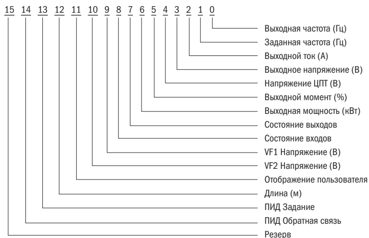
Рисунок 43 — Отображение 1 LED при работе
