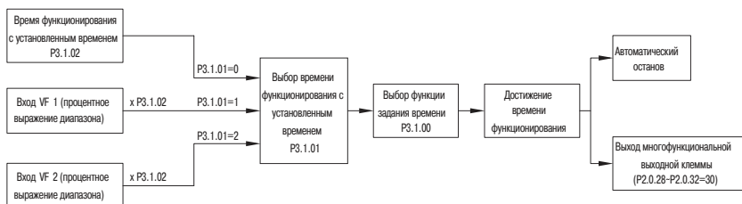
Рисунок 61 — Работа функции контроля времени
