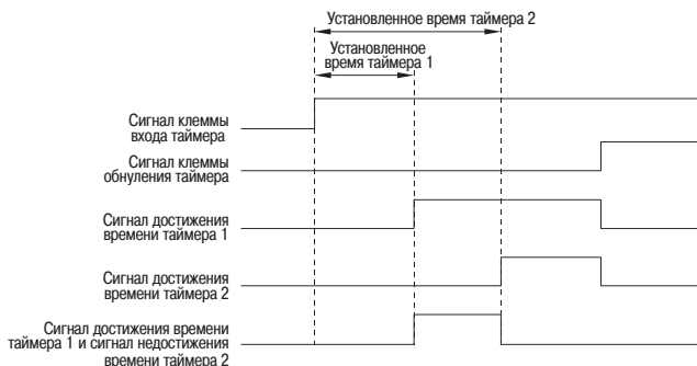
Рисунок 72 — Обнуление таймеров
