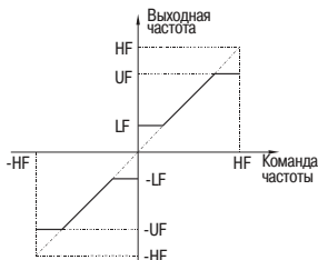
Рисунок 25 — Пределы частоты
