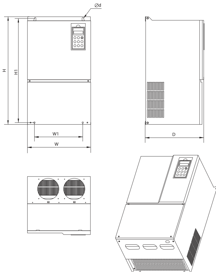
Габарит 5.2
