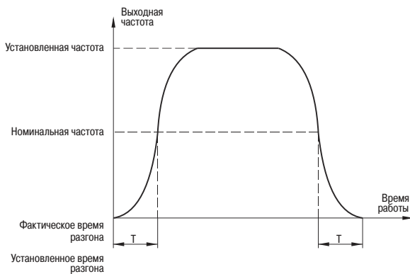
Рисунок 27 — S кривая ускорения и замедления
