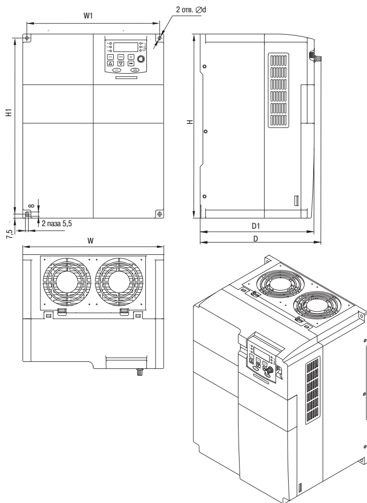
Габарит 5
