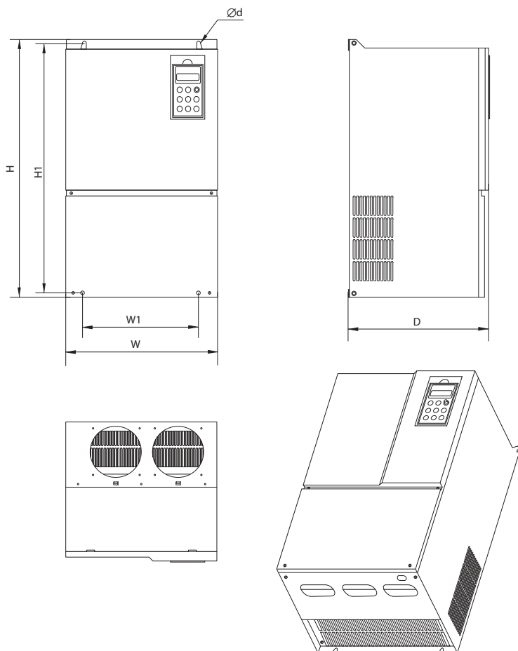
Габарит 5.1
