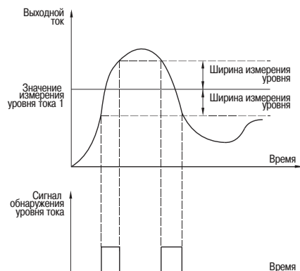
Рисунок 40 — Измерение уровня тока
