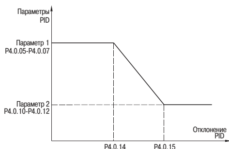
Рисунок 41 — Переключение ПИД
