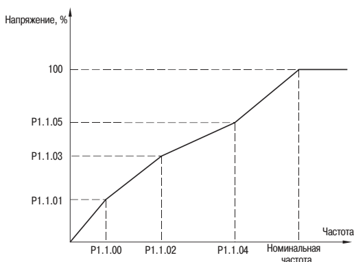
Рисунок 33 — Произвольная кривая V/F
