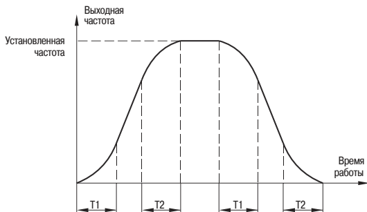
Рисунок 28 — Соотношения S кривых
