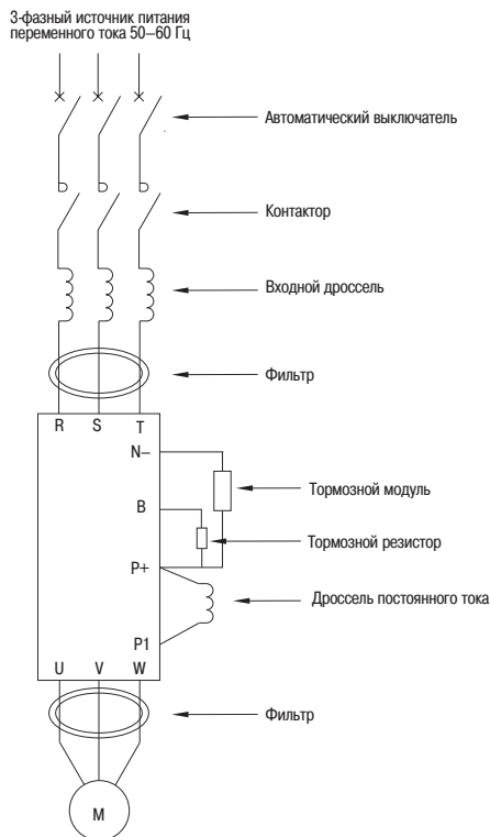
Рисунок 8 – Подключение периферийных устройств
