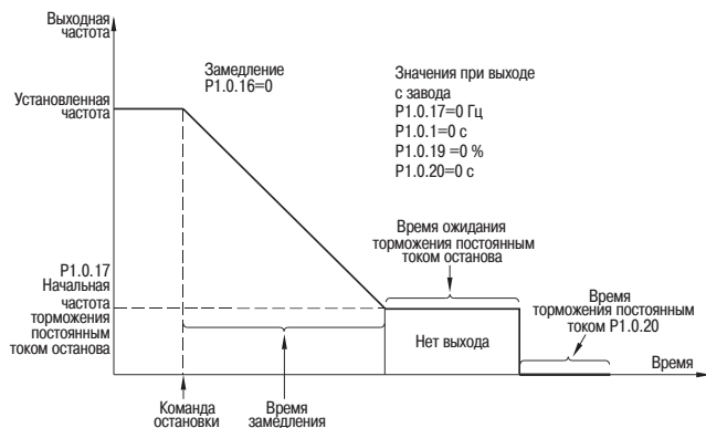
Рисунок 56 — Остановка замедлением
