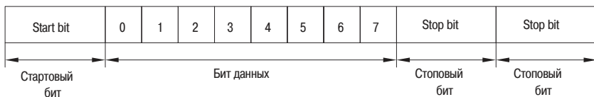
Рисунок 83 – 8-N-2, P4.1.01 = 0
