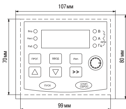
Рисунок 21 — Габаритные размеры пульта управления
