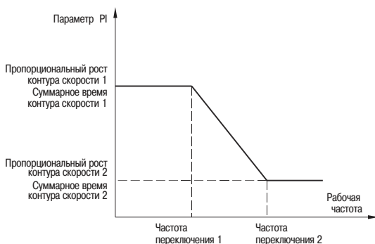
Рисунок 31 — Частоты переключения
