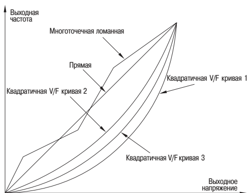
Рисунок 30 — V/F-кривые
