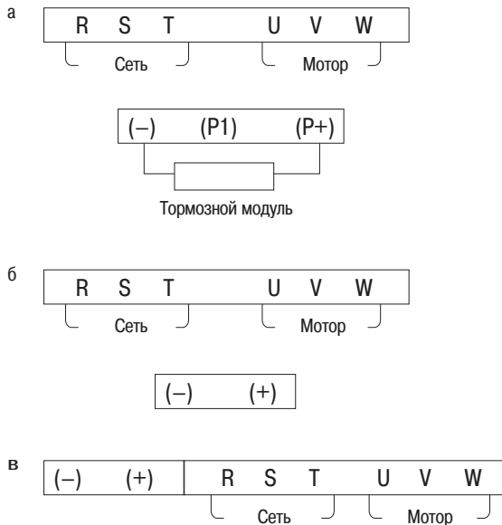
Рисунок 11 — Схема подключения силовой цепи преобразователей: а) габарит 9, б) габариты 10, 11 и 12, в) габарит 13
