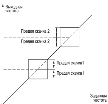
Рисунок 29 — Скачкообразные частоты
