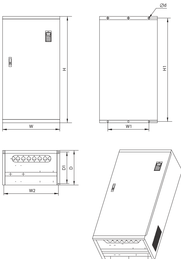
Габарит 5.4
