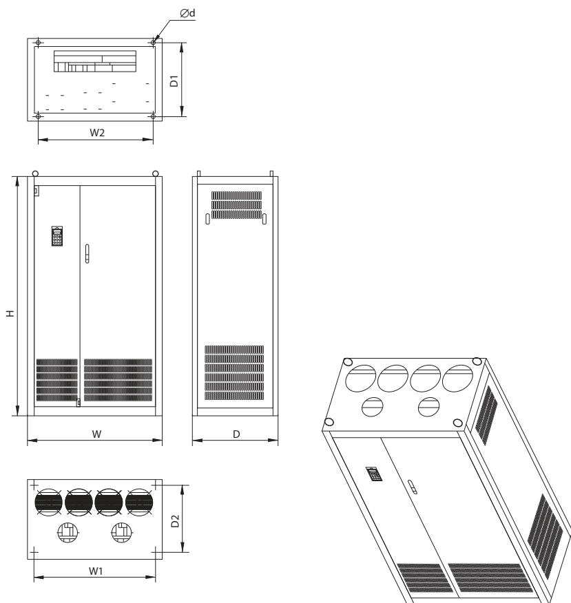
Габарит 5.8
