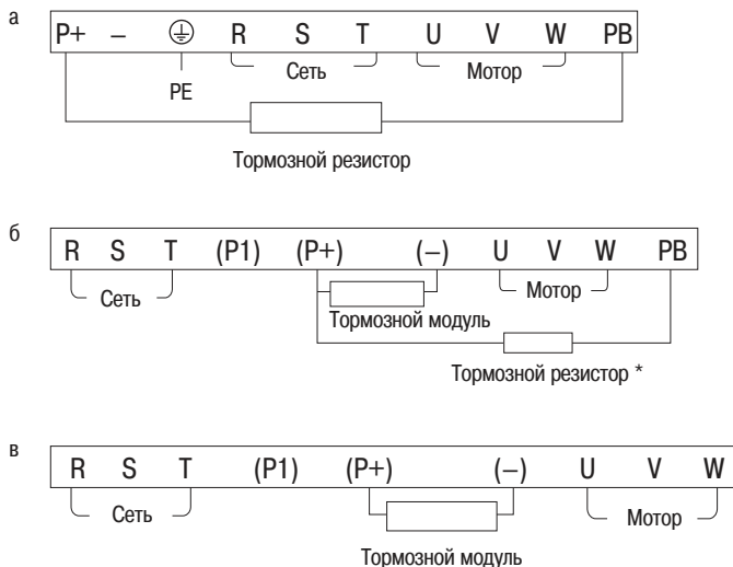
Рисунок 10 — Схема подключения силовой цепи преобразователей: а) габариты 3, 4 и 5, б) габарит 6, в) габариты 7 и 8
