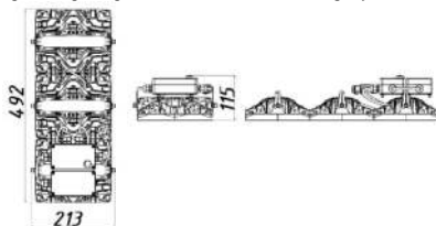
Рисунок 1 Общий вид светильника «L-pixel 3 Em» Подвесное крепление
