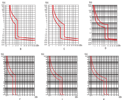
Рис. 1 Время-токовые характеристики
