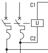
Схема подключения
