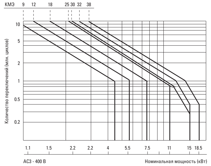
Рис. 1 – Коммутационная износостойкость контакторов КМЭ 9-38 А
