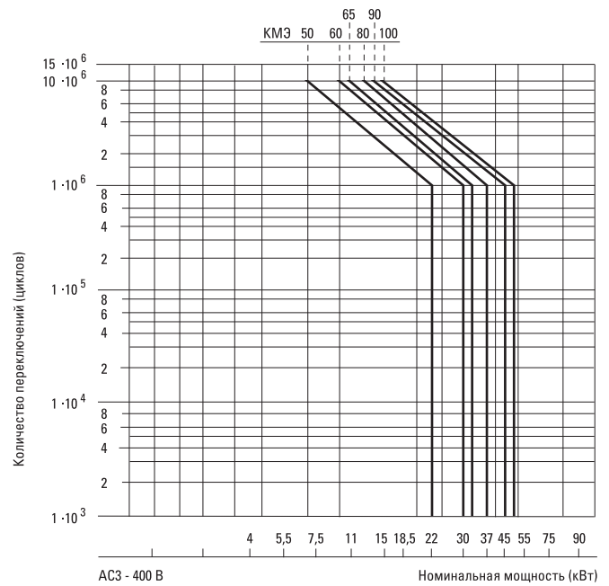
Рис. 2 – Коммутационная износостойкость контакторов КМЭ 50-100 А
