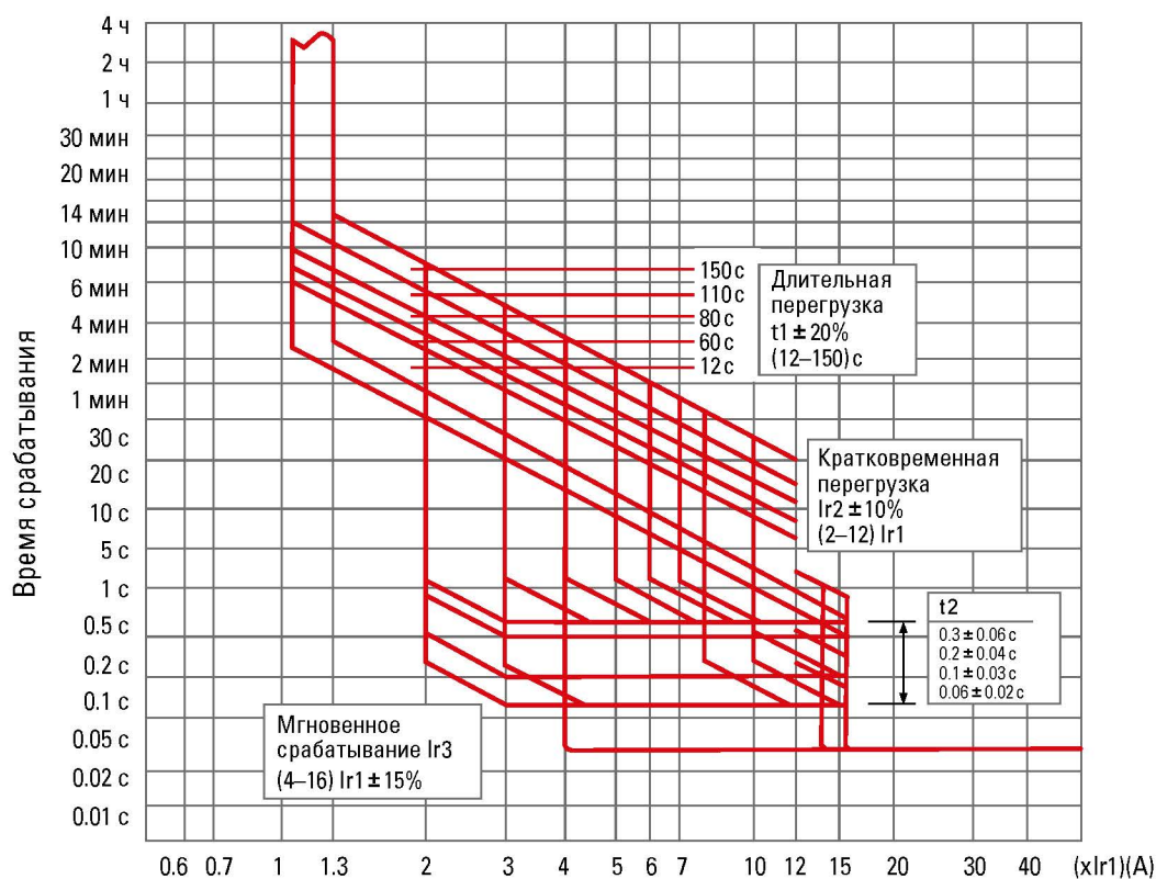
BA-99M/ 63-800 А с электронным расцепителем
