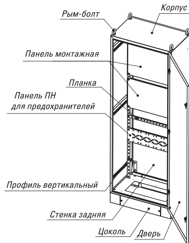
Рис.1. Схема монтажа
