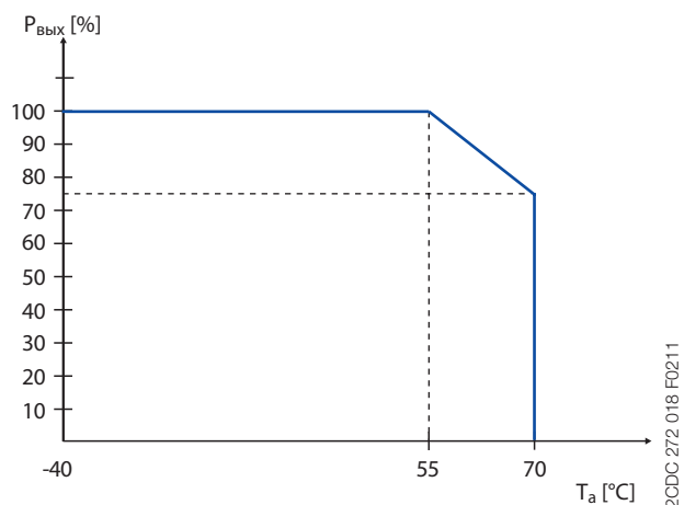
CP-E 24/20.0, CP-E 48/10.0
