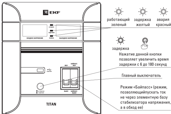
Рис. 4 Внешний вид стабилизатора F-3000-5000
