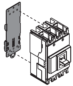
Скоба для DIN-рейки для 3 п. автоматического выключателя
