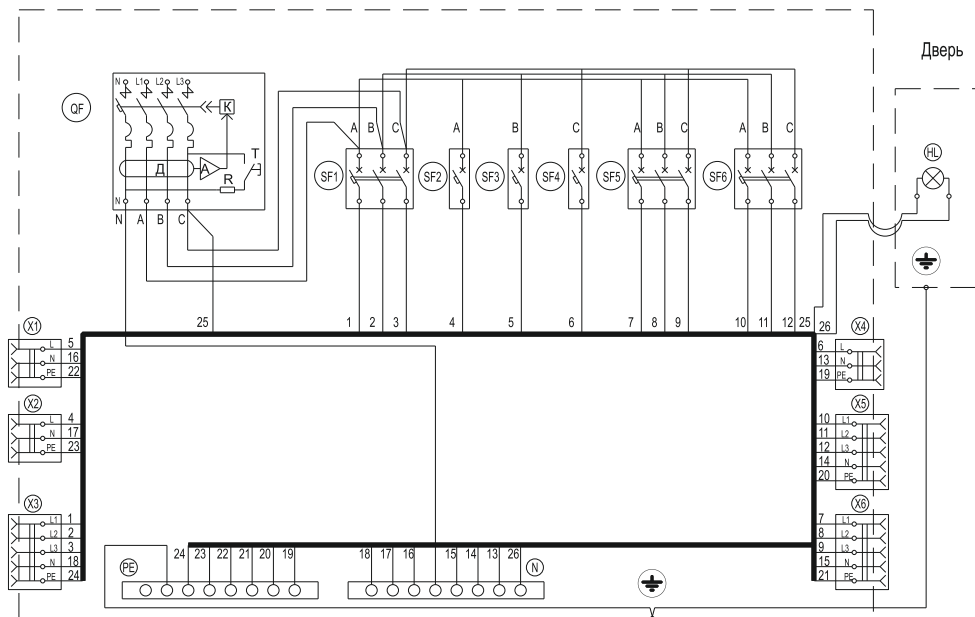
Рисунок 1 – Схема электрическая
