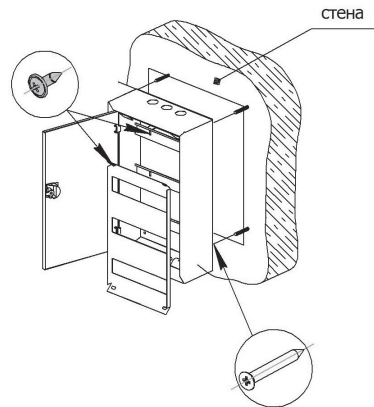
Рис.1. Схема монтажа
