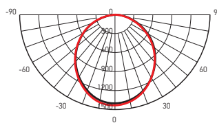
PPL PRO 595/U Opal 36w
