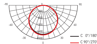
PPL PRO 595/U Prisma 36w
