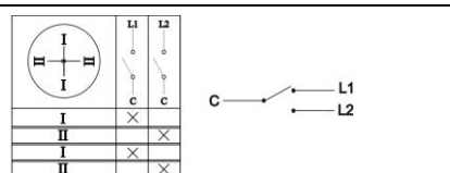
Рисунок 17. Пакетный переключатель 1-полюсный 4С
