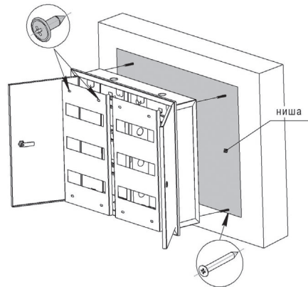
Рис.1. Схема монтажа
