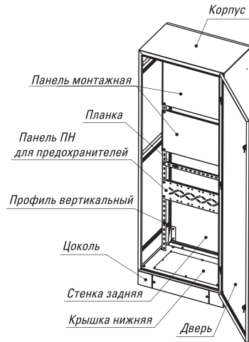
Рис.1. Схема монтажа
